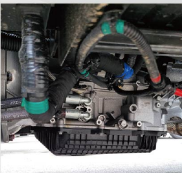
직결형 PTO ※드라이브샤프트 없음!
